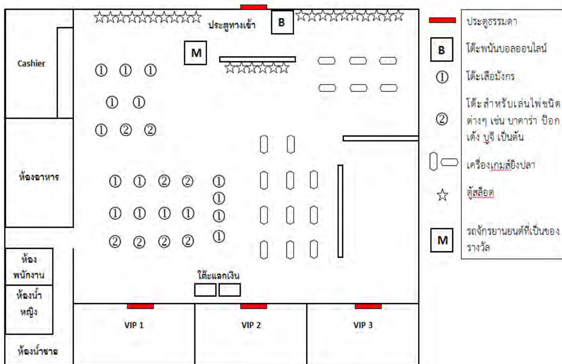
ภาพที่ 45 ภาพแผนผังคาสิโนชั้น ซิตี
